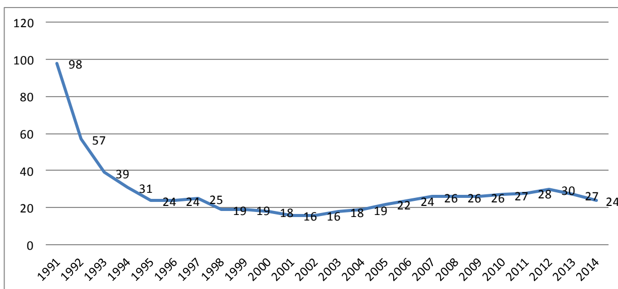
Рисунок 1. Добыча нефти в 1991-2014 годах в Таджикистане. На горизонтальной оси представлено время, а на вертикальной оси-объемы добычи в тысячах тонн.
